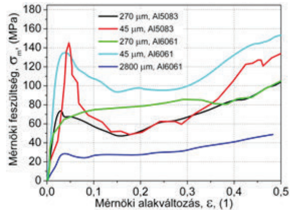
5. ábra Al5083 és Al6061 szintaktikus habok nyomófeszültség-alakváltozás görbéi, Palmer és társai nyomán [33]
