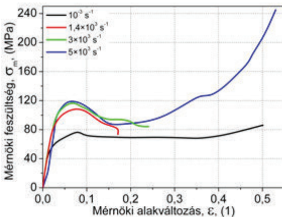
9. ábra 90 \mu\text{m} -es (balra) és 150 \mu\text{m} -es (jobbra) átlagos gömhéj átmérővel rendelkező szintaktikus habok statisztikus- és dinamikus körülmények között rögzített mérnöki feszültség-mérnöki alakváltozás diagramjai, Dou és társai nyomán [63]
