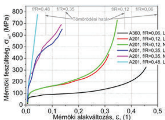
11. ábra Radiális irányban gátolt alakváltozású próbatestek mérnöki feszültség – mérnöki alakváltozás diagramjai (L=lágyított, N=nemesített), Kiser és társai nyomán [105]
